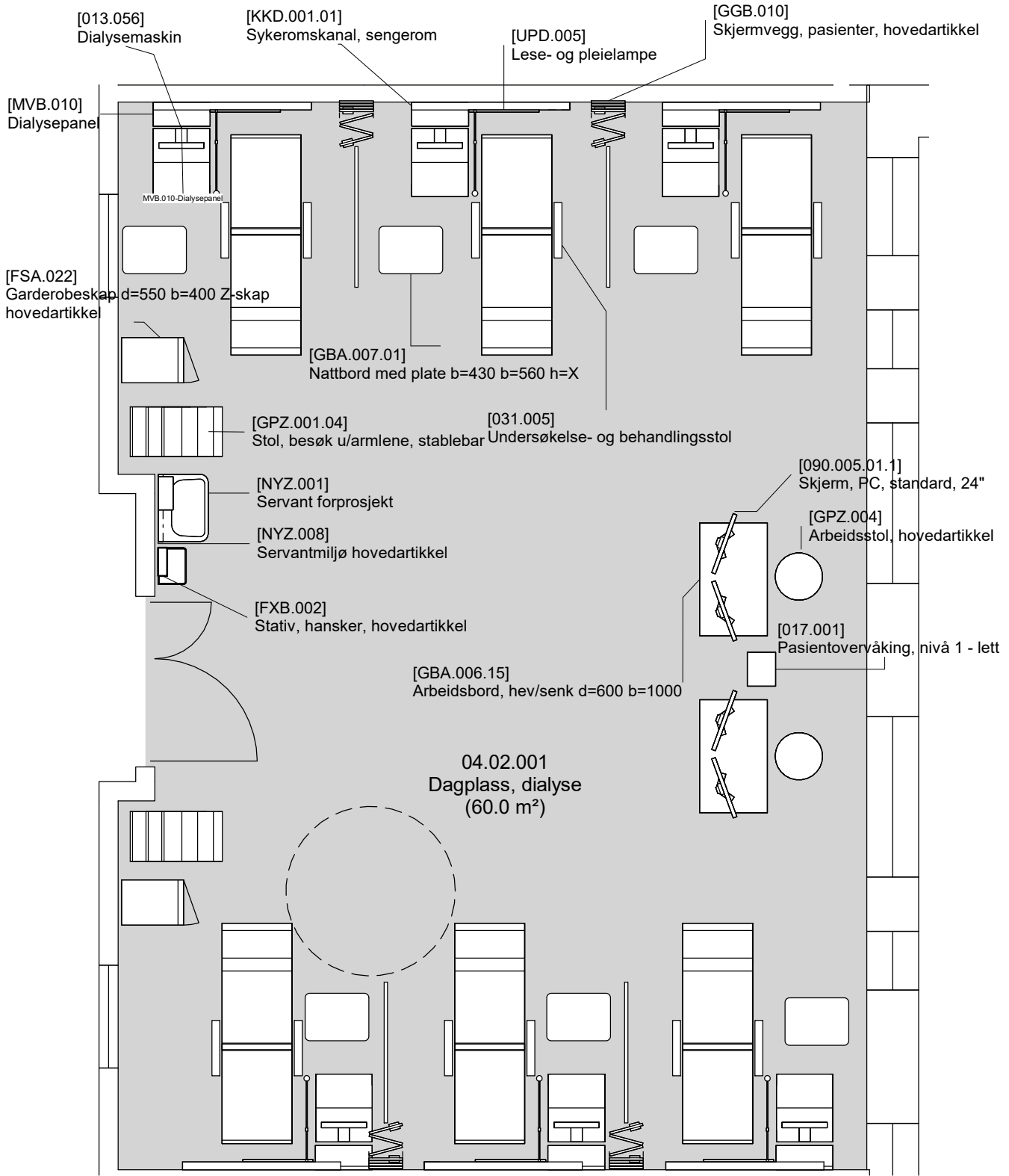
Planutsnitt 04.02.001 Dagplass, Dialyse
